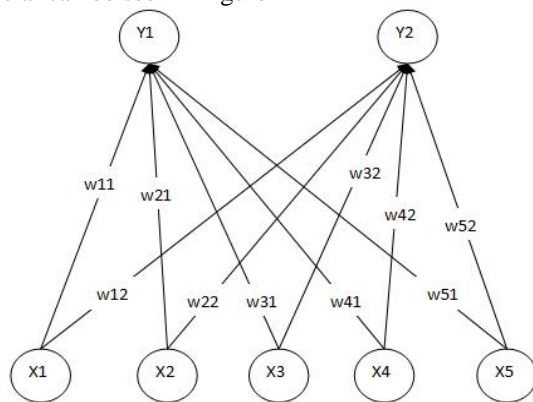
Figure 2 : SOM Architecture
